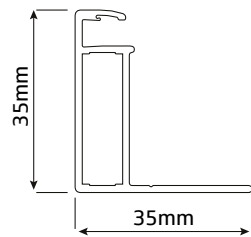
Rahmenprofil
